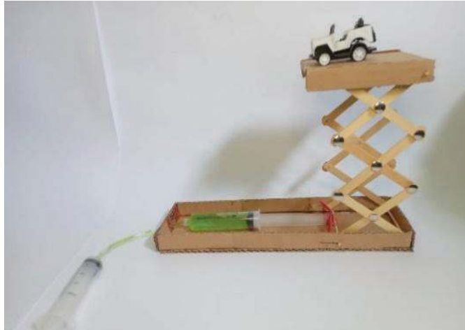
Gambar 4.1 Miniatur dongkrak hidrolik Sumber: Novi Nurhayati (2022)
